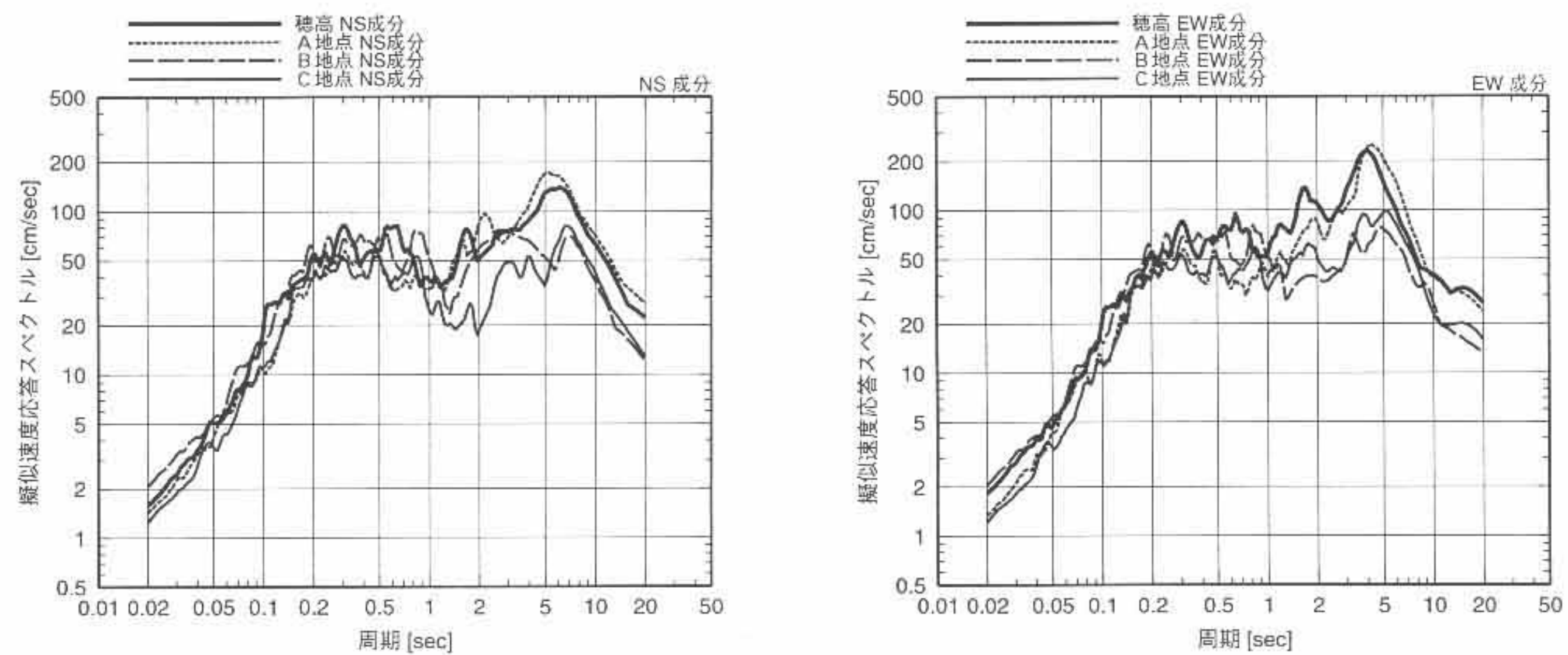
図15 試算結果による擬似速度応答スペクトル (減衰定数5%) の比較
