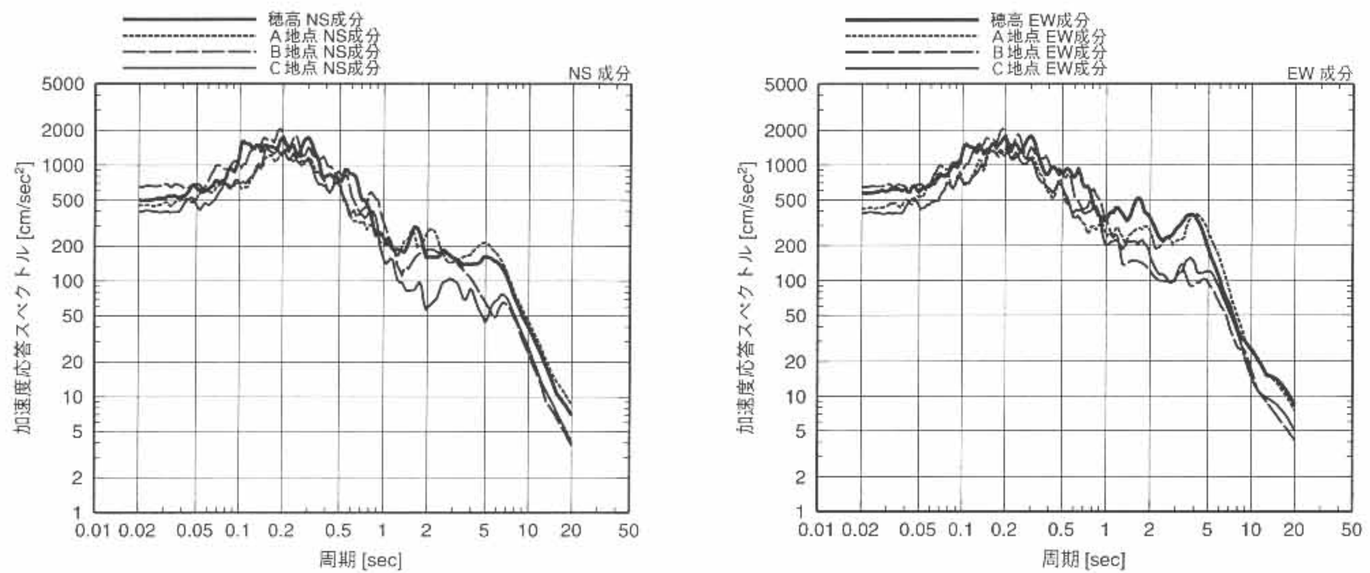
図14 試算結果による加速度応答スペクトル (減衰定数5%) の比較
