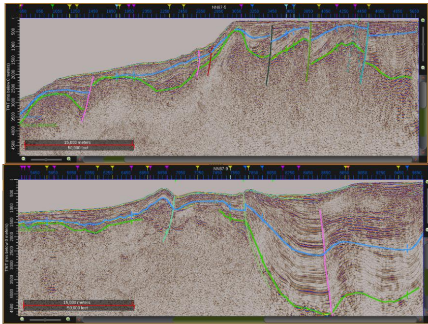
男鹿半島周辺の震探断面図。(上)北側、(下)南側。
