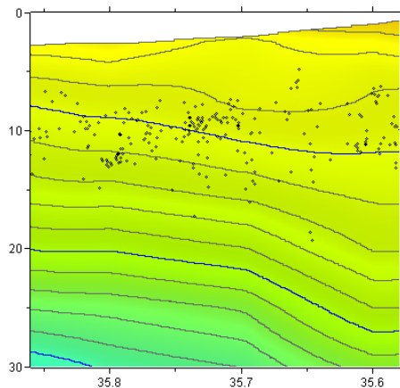
図 17-4 浦底-柳ヶ瀬山断層帯に平行及び直交する断面の震源分布図
