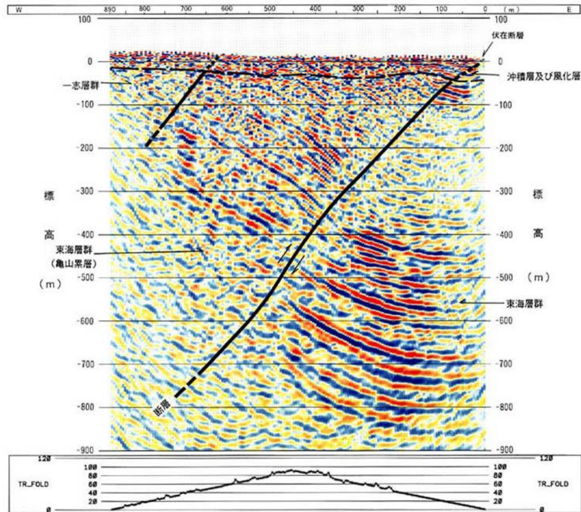
図4 反射法地震探査片田測線の解釈断面図（三重県，1998）
