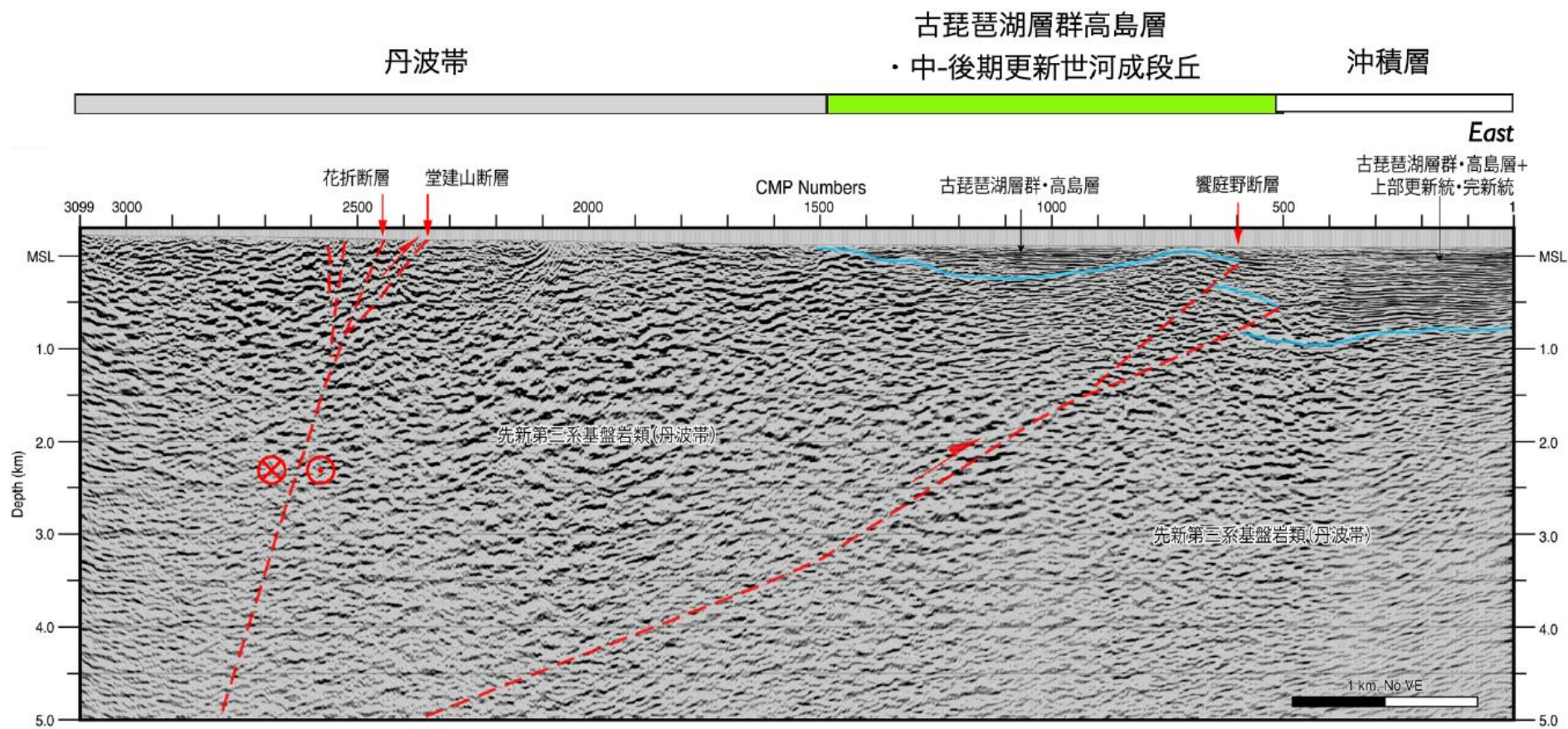
図4 響庭野-朽木測線の反射法弾性波探査断面（図2のB測線） （文部科学省研究開発局・国立大学法人東京大学地震研究所，2020）
