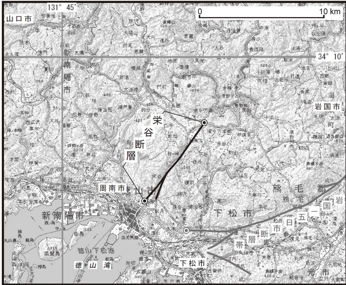
図1 栄谷断層の位置
