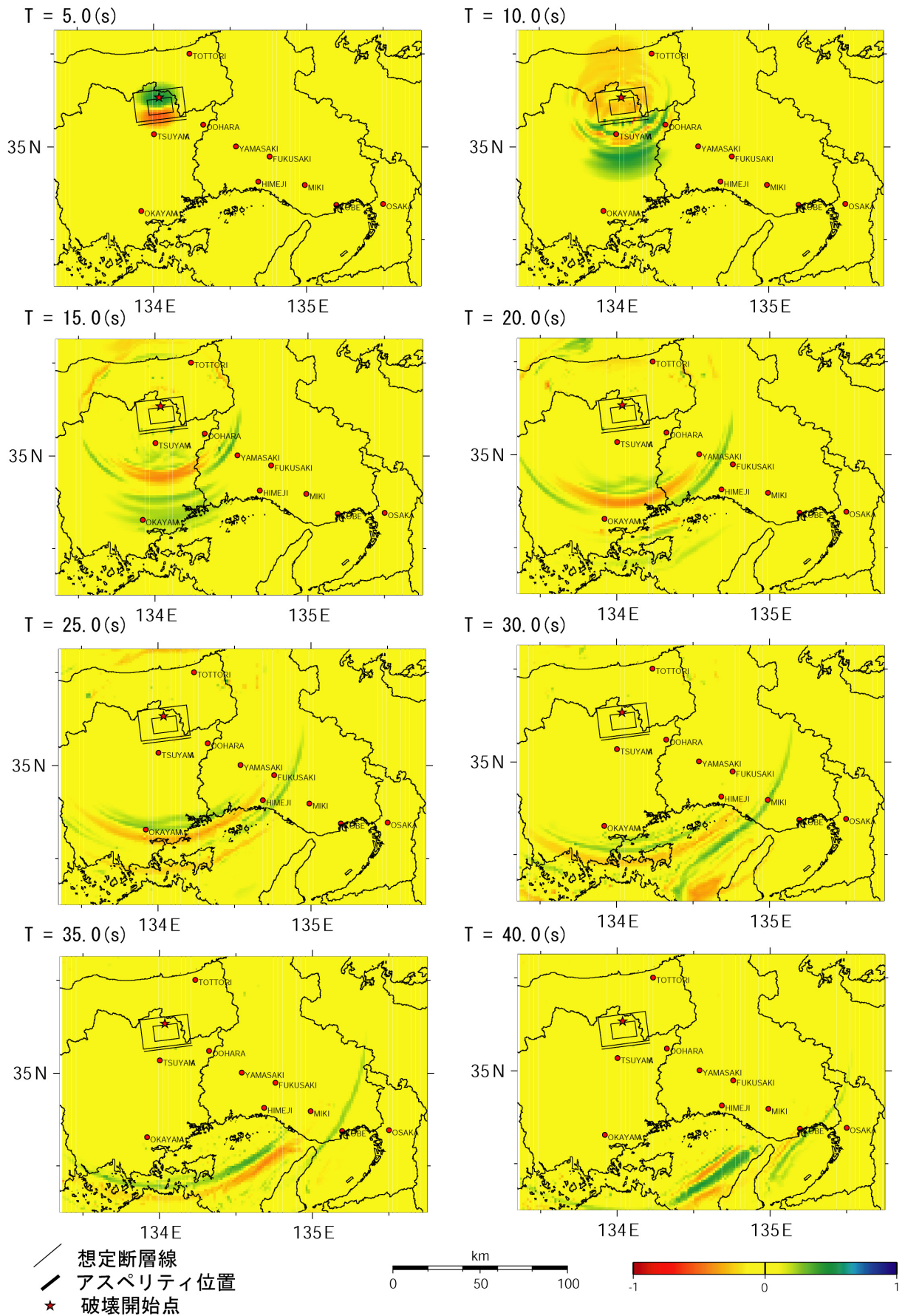
図 15-6 有限差分法による計算結果例 (モデル5、「詳細法工学的基盤」 ( V_s=550\text{m/s} 、 V_s=590\text{m/s} ) 上の速度振幅のスナップショット、NS 成分)
