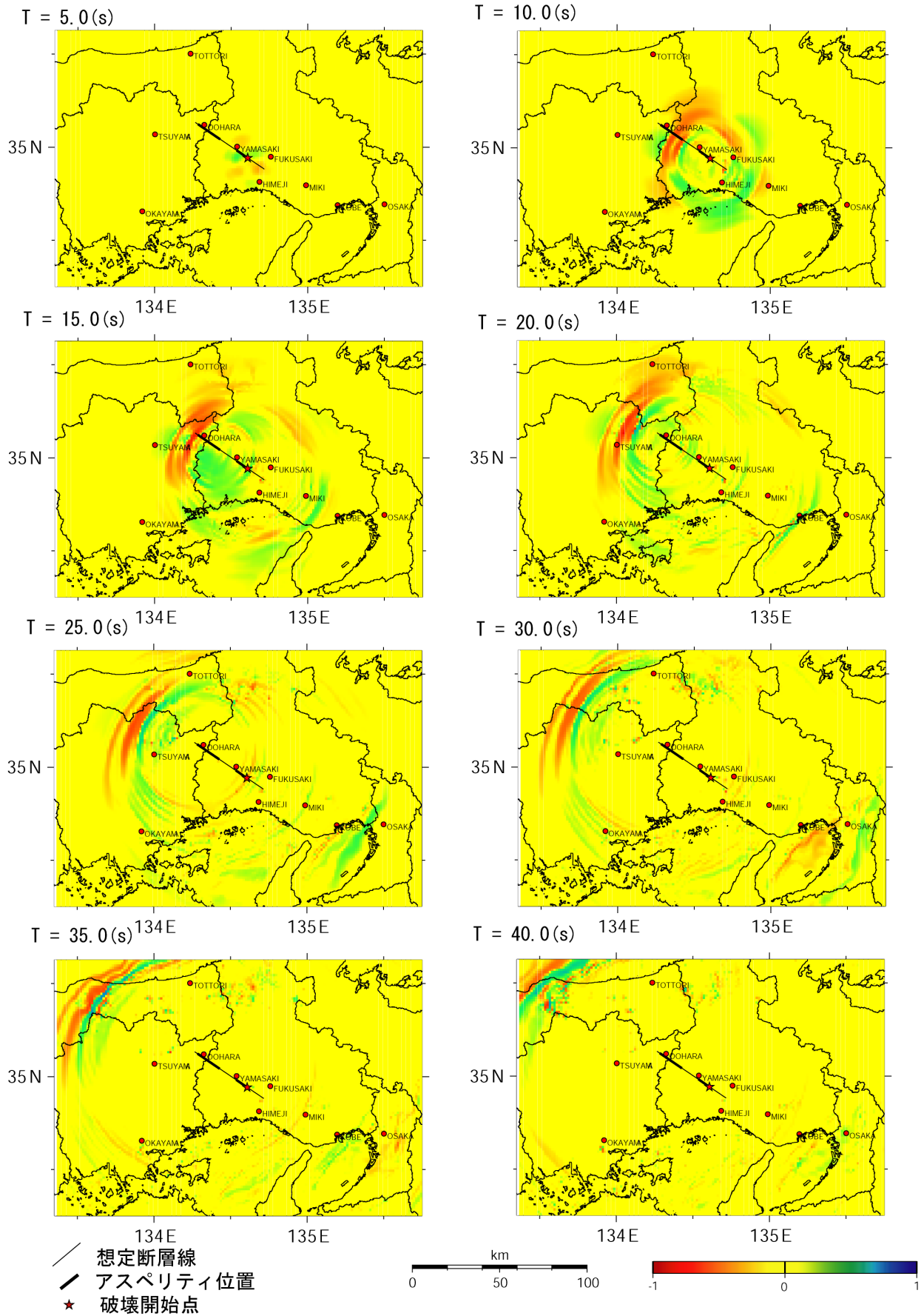
図 1 5 - 3 有限差分法による計算結果例 (モデル 2 : ケース 2 - 2、「詳細法工学的基盤」 ( V_s=550\text{m/s} 、 V_s=590\text{m/s} ) 上の速度振幅のスナップショット、NS 成分)
