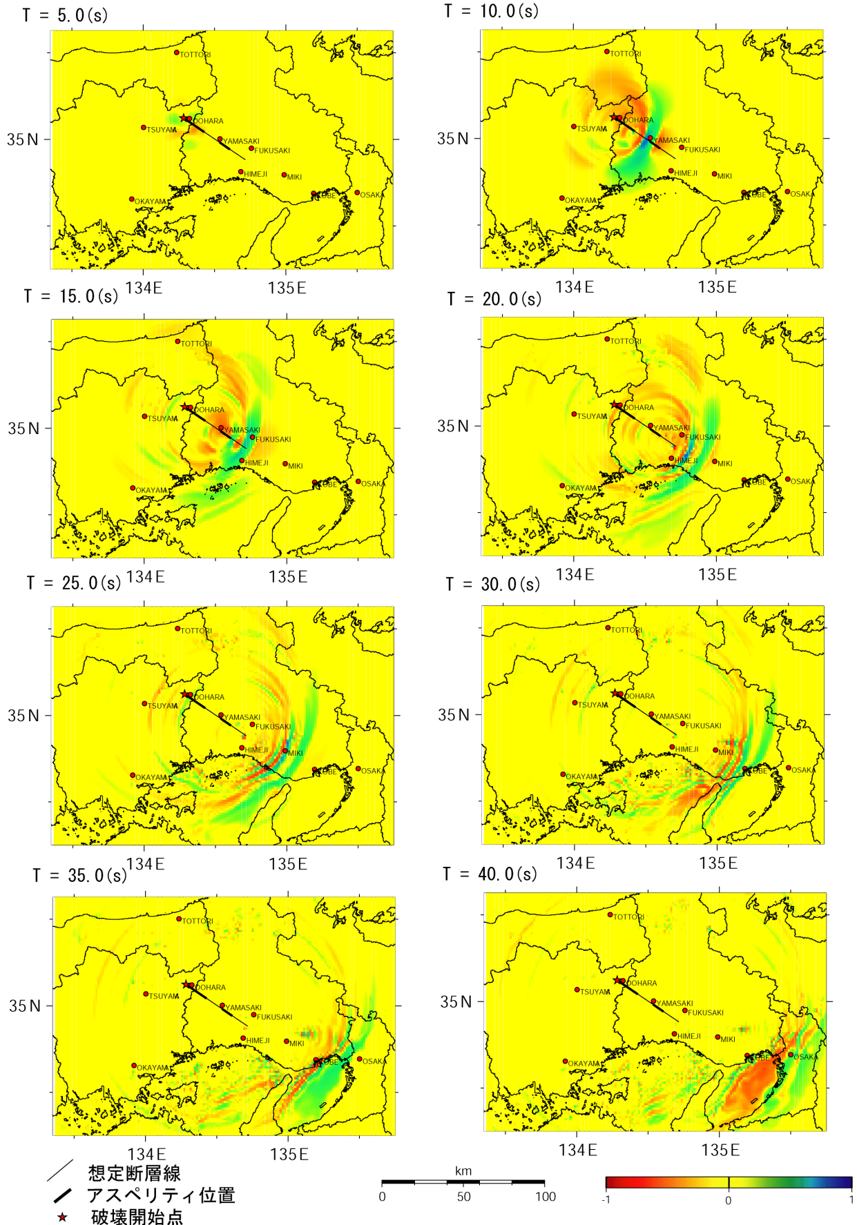
図 1 5 - 2 有限差分法による計算結果例 (モデル 2 : ケース 2 - 1、「詳細法工学的基盤」 ( V_s=550\text{m/s} 、 V_s=590\text{m/s} ) 上の速度振幅のスナップショット、NS 成分)
