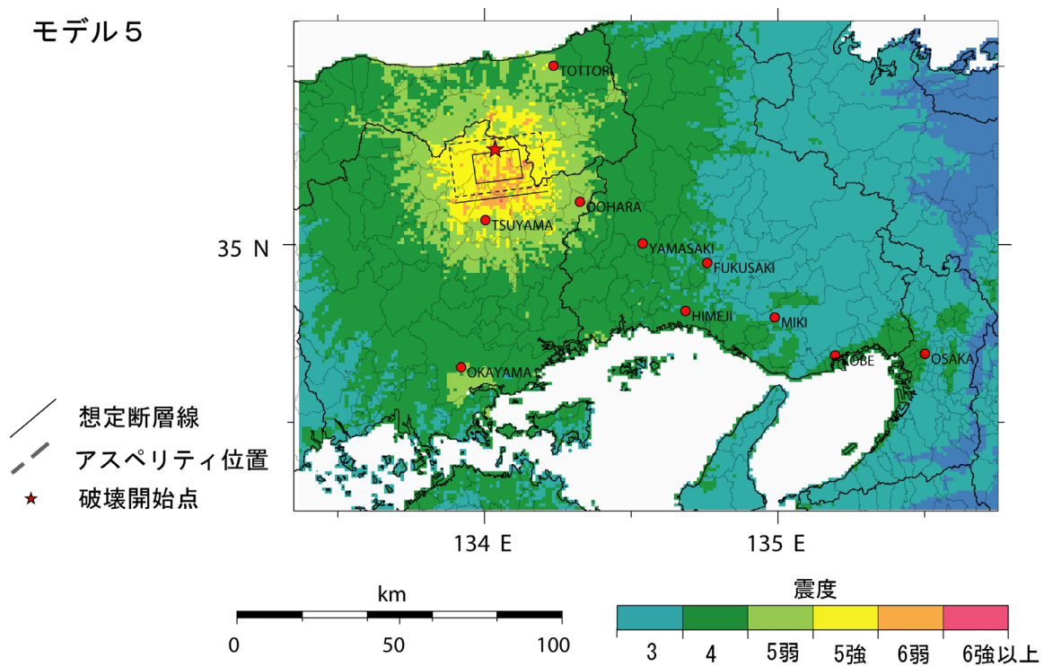
図5-4 詳細法による強震動予測結果：地表の震度分布（モデル5）
