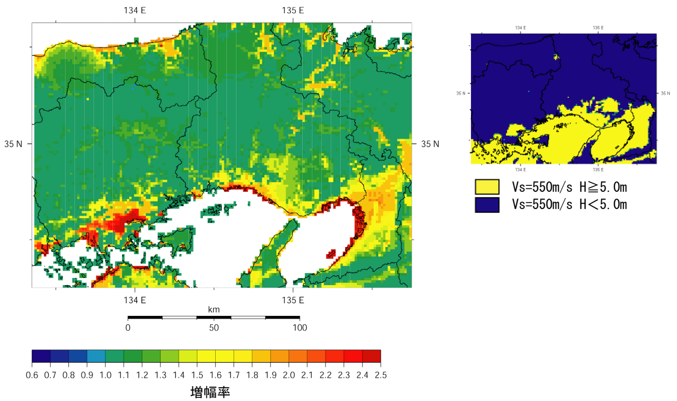
図4 「詳細法工学的基盤」( V_s=550\text{m/s} の層厚が5 m以上の場合は V_s=550\text{m/s} 、5 m未満の場合は V_s=590\text{m/s} とする。(右図参照)) から地表までの最大速度の増幅率(「浅い地盤構造」)
