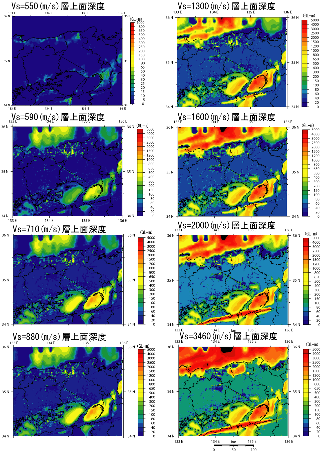
図3 「深い地盤構造」に用いた三次元地下構造モデル (各速度層上面の深さ分布[GLm])
