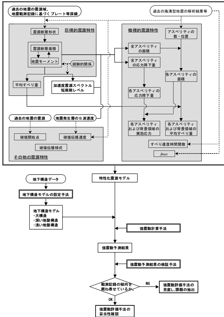
図 2.2.2-1 海溝型地震の強震動予測手法の検証の流れ
