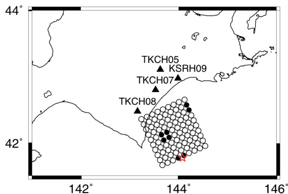
図 2. 2. 6-3(2) 平成 15 年 (2003 年) 十勝沖地震の観測波形記録と 詳細法による計算波形との比較例 (つづき: 震源域に近い観測点)
