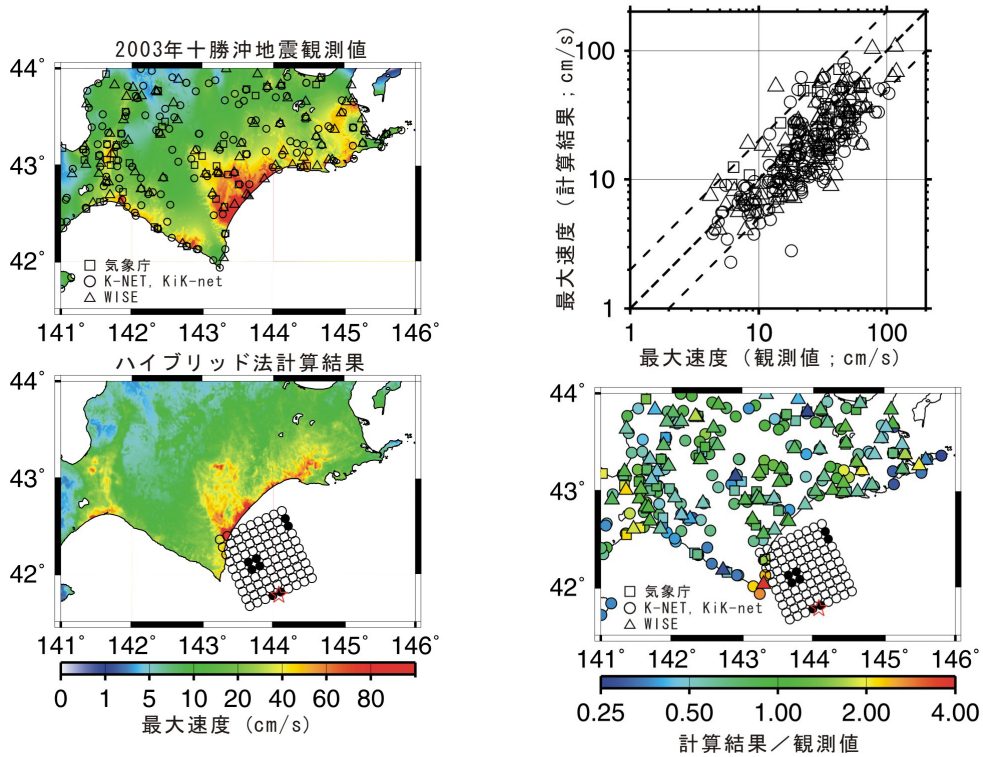
図 2.2.6-8(1) ハイブリッド合成法による強震動計算結果と平成 15 年（2003 年）十勝沖地震の観測記録との比較（地表の最大速度分布の比較。観測記録のコンター図（左上図）は、図 2.2.6-2 と同様の方法により作成した。）
