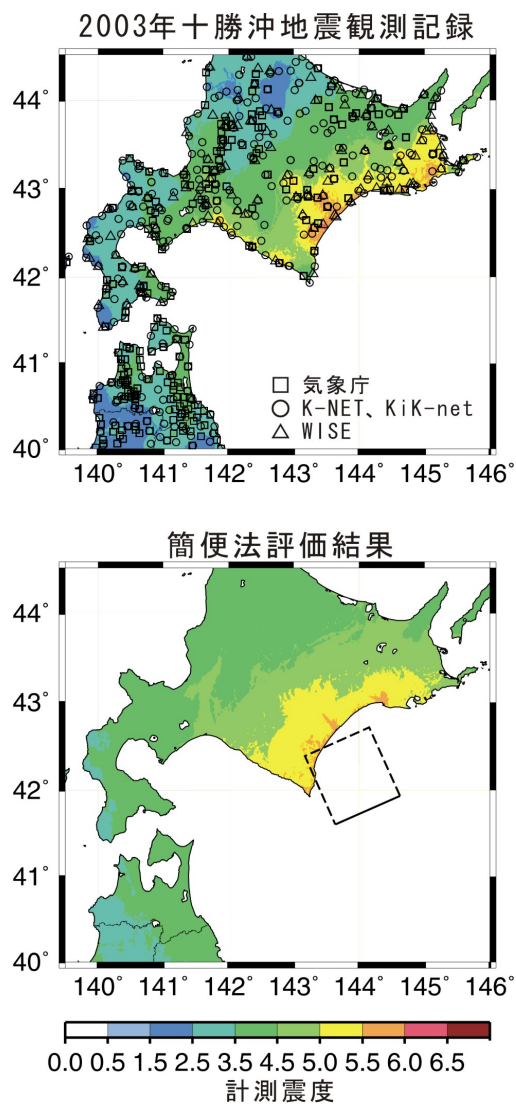
図 2.2.6-9 簡便法による強震動予測結果と観測された震度との比較 (観測記録のコンター図(上図)は、図 2.2.6-2 と同様の方法により作成した。)
