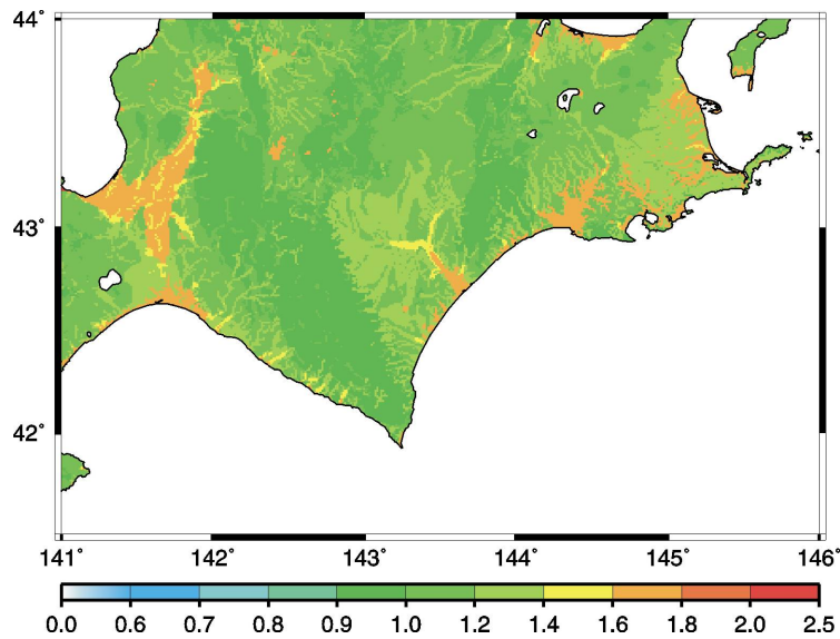
図 2. 2. 4-4 「詳細法工学的基盤」(Vs=480m/s) から地表までの最大速度の地盤増幅率分布（「浅い地盤構造」、藤本・翠川, 2003）
