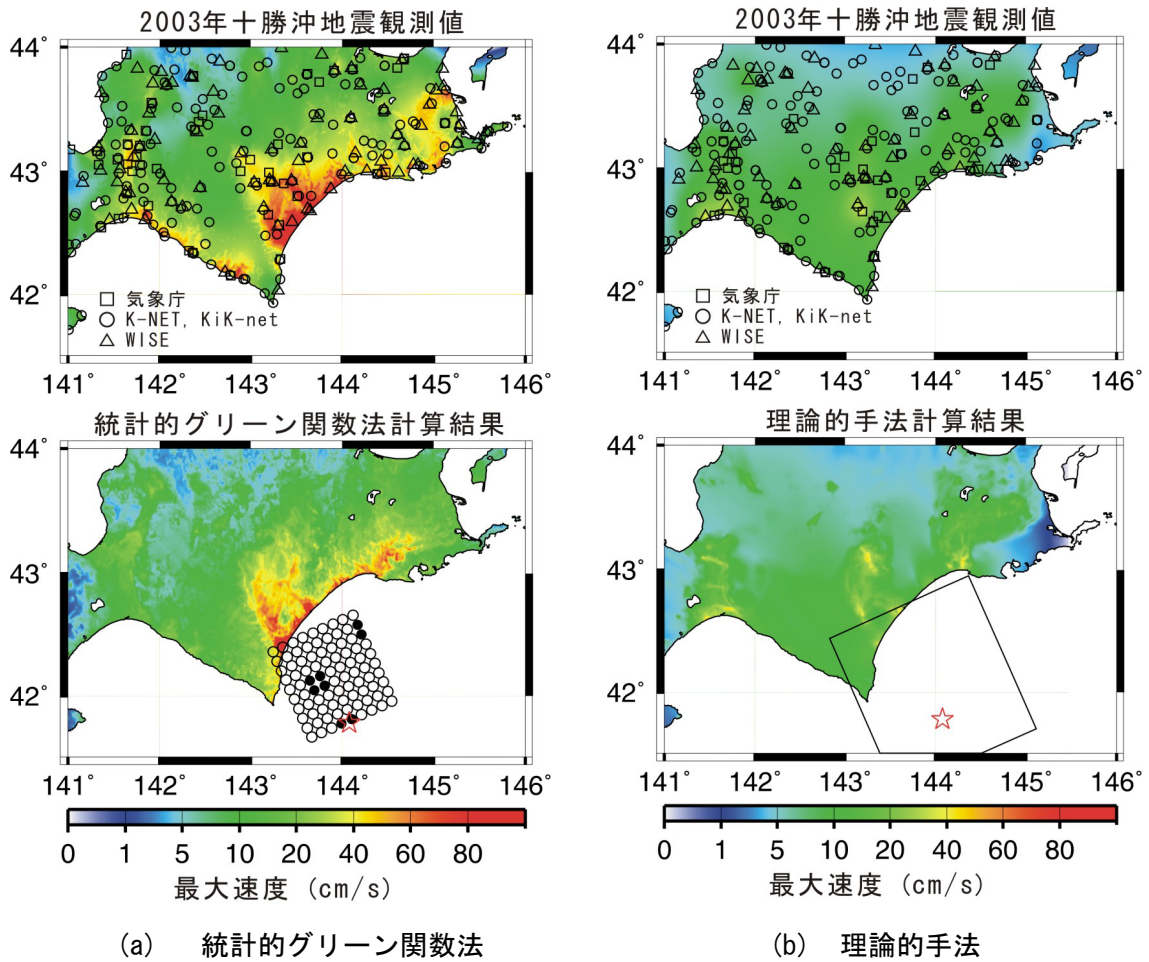
図 2.2.6-2 観測記録と詳細法（統計的グリーン関数法、理論的手法）による強震動評価結果の比較（地表の最大速度分布。観測記録のコンター図（上図）は、地表の最大速度を藤本・翠川（2003）による工学的基盤から地表までの最大速度の増幅率で除して、工学的基盤上の最大速度に換算し、工学的基盤上でコンターを作成した後、このコンターに最大速度の増幅率を再度乗じることにより作成した。）
