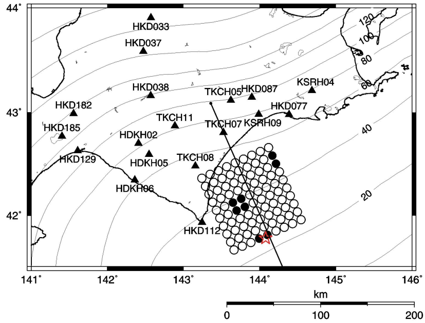
図 2.2.2-3 「詳細法」による平成 15 年（2003 年）十勝沖地震の強震動評価対象領域と震源断層モデル（●はアスペリティ、☆は破壊開始点）
