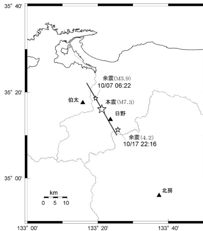
図2.1.3-1 鳥取県西部地震の震源断層（太線）と試算地点（▲）位置図
