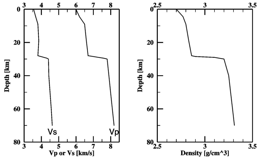
図 2.2.4-1 Iwasaki et al. (1991)に基づく、「詳細法」の理論的手法による計算に用いた上部マントルから地震基盤までの大構造モデル (左: P 波速度および S 波速度、右: 密度)
