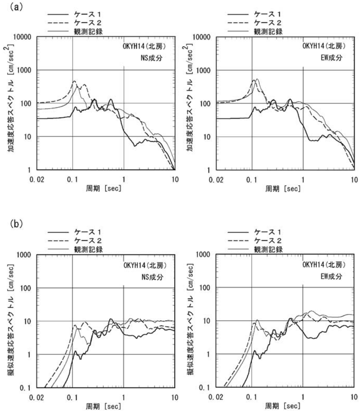
図2.1.3-4(3) 地中観測点におけるスペクトル（観測波形、ケース1、ケース2）の比較 （北房観測点；（a）：5%減衰加速度応答スペクトル （b）：5%減衰擬似速度応答スペクトル）
