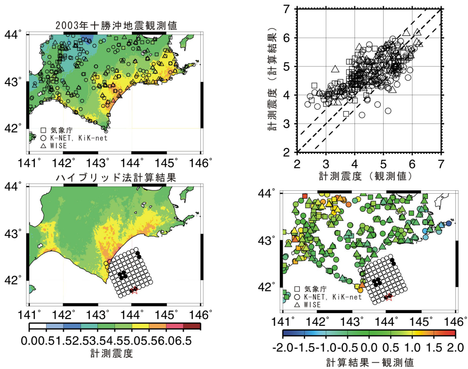
図 2.2.6-8(2) ハイブリッド合成法による強震動計算結果と平成 15 年（2003 年）十勝沖地震の観測記録との比較（計測震度分布の比較。観測記録のコンター図（左上図）は、図 2.2.6-2 と同様の方法により作成した。）
