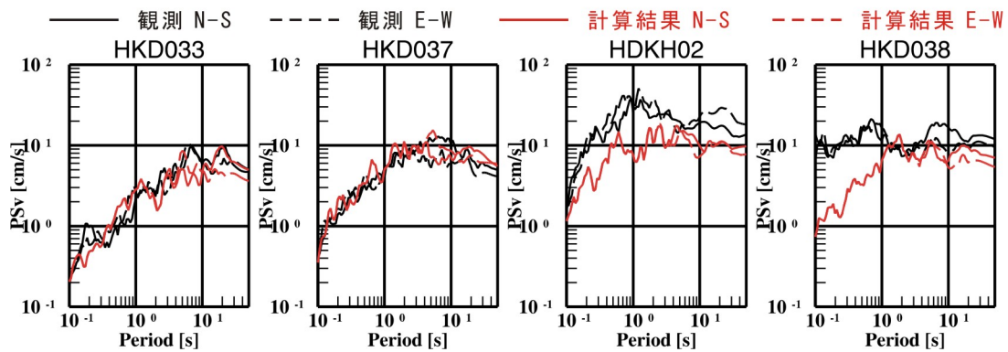
図 2.2.6-6 図 2.2.6-3(4)に示した観測点における観測波形記録と詳細法による計算波形との比較 (減衰特性 (Q値)を変えた検討)
