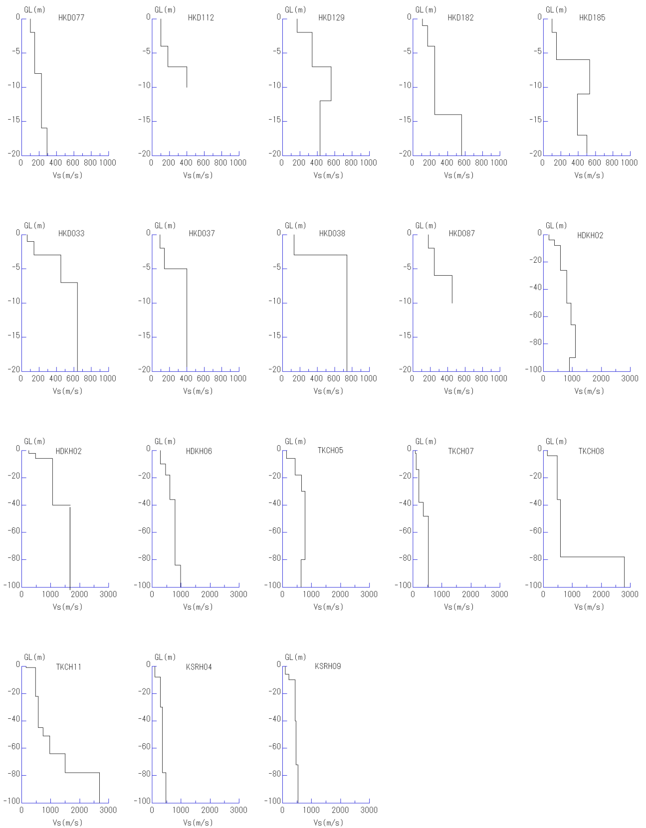
図 2.2.4-5 地表における波形の計算に用いた各観測点の一次元地下構造 (S 波速度)
