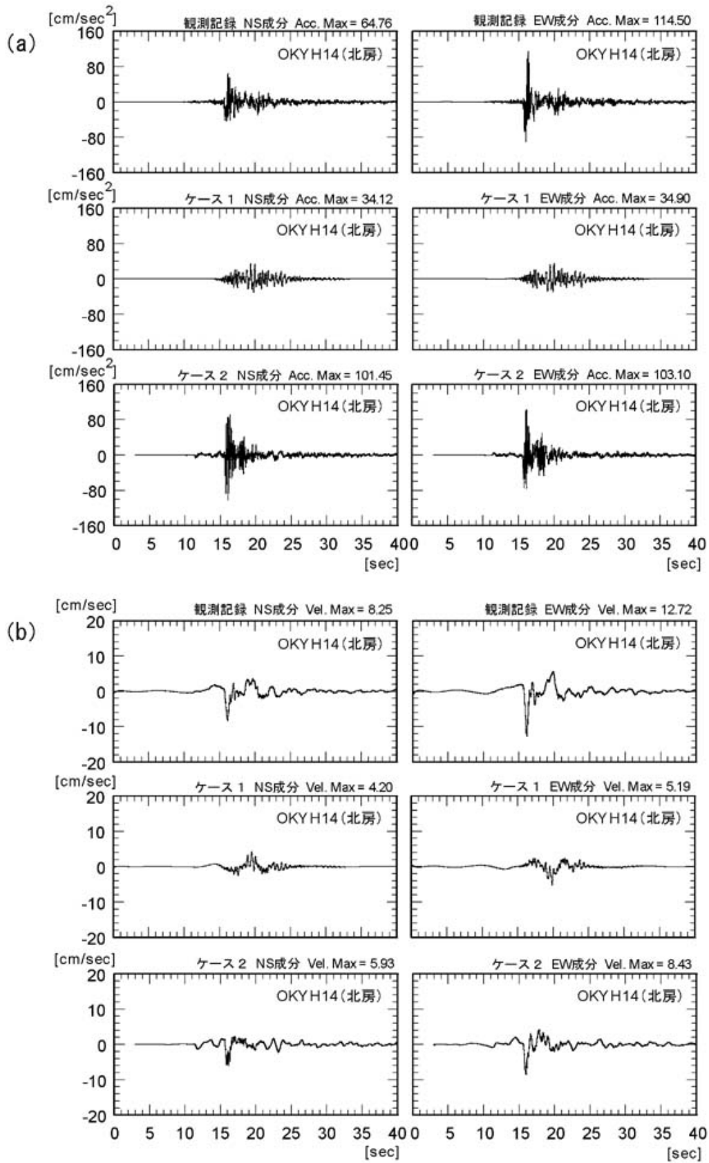
図2.1.3-3(3) 地中観測点における地震波形（観測波形、ケース1、ケース2）の比較（北房観測点；（a）：加速度波形 （b）：速度波形）
