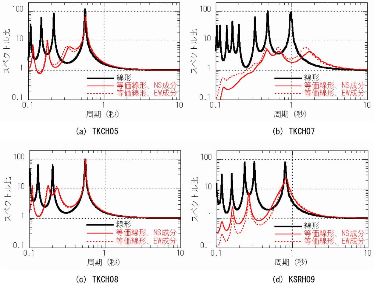
図 2.2.6-5 各 KiK-net 観測点における孔中と地表でのスペクトル比の比較 (黒：線形、赤：等価線形 (実線：NS、点線：EW))
