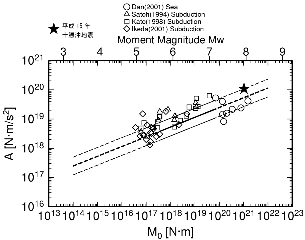
図 2.2.3-1 平成 15 年（2003 年）十勝沖地震の短周期レベルと地震モーメントの関係（壇ほか，2001 に加筆）
