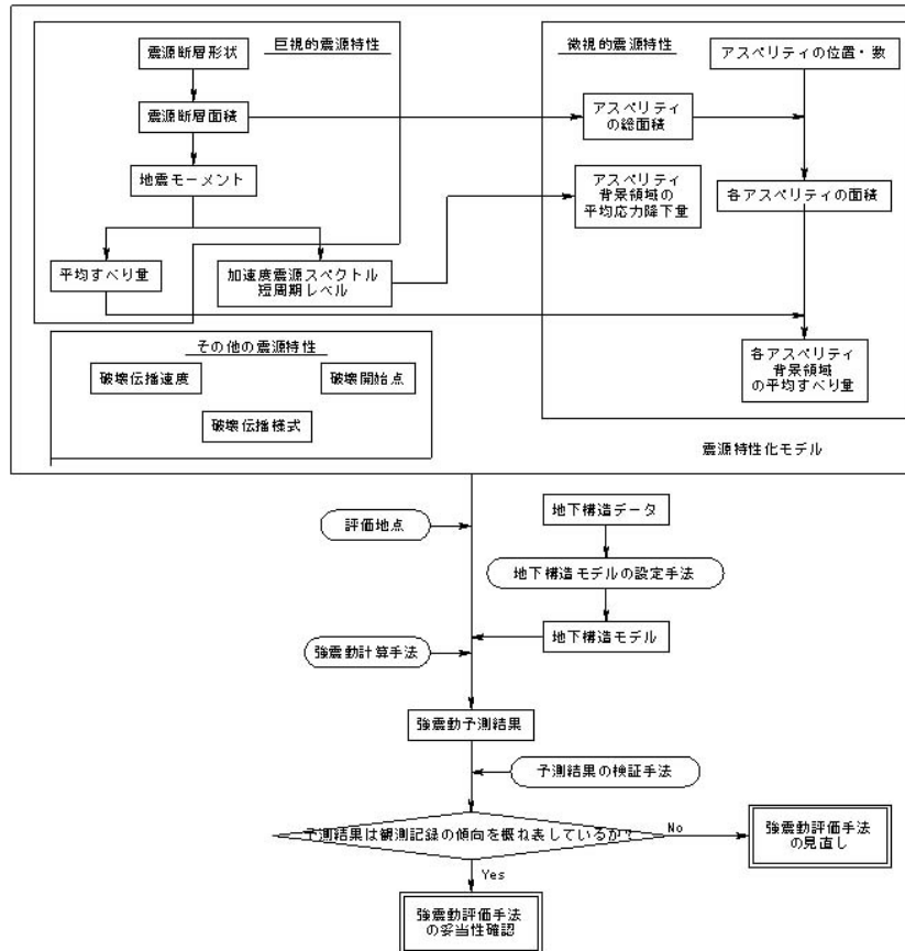
図2.1-1 鳥取県西部地震の観測記録を利用した強震動予測手法の検証の流れ
