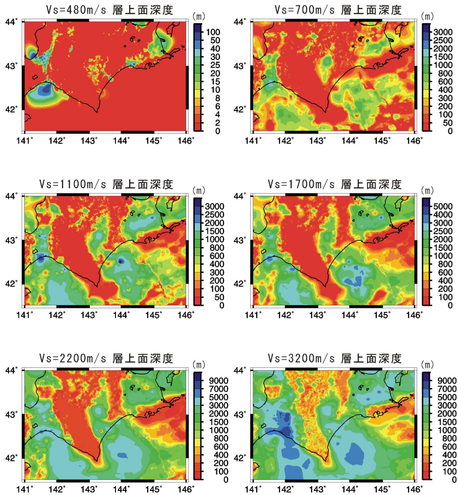
図 2. 2. 4-3 「深い地盤構造」に用いた三次元地下構造モデル（各速度層上面の深さ分布）
