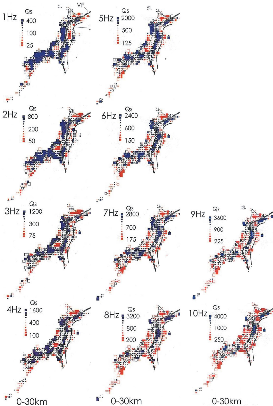
図 2.2.6-7 三次元 Q 構造 (中村・植竹, 2002 より深さ 0-30km のみ抜粋)
