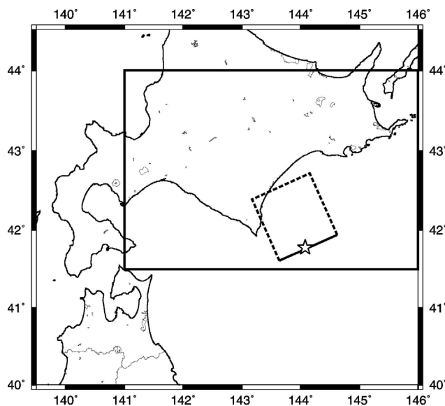
図 2.2.2-2 断層面の設定位置と簡便法の計算領域および詳細法の計算領域（太線枠）
