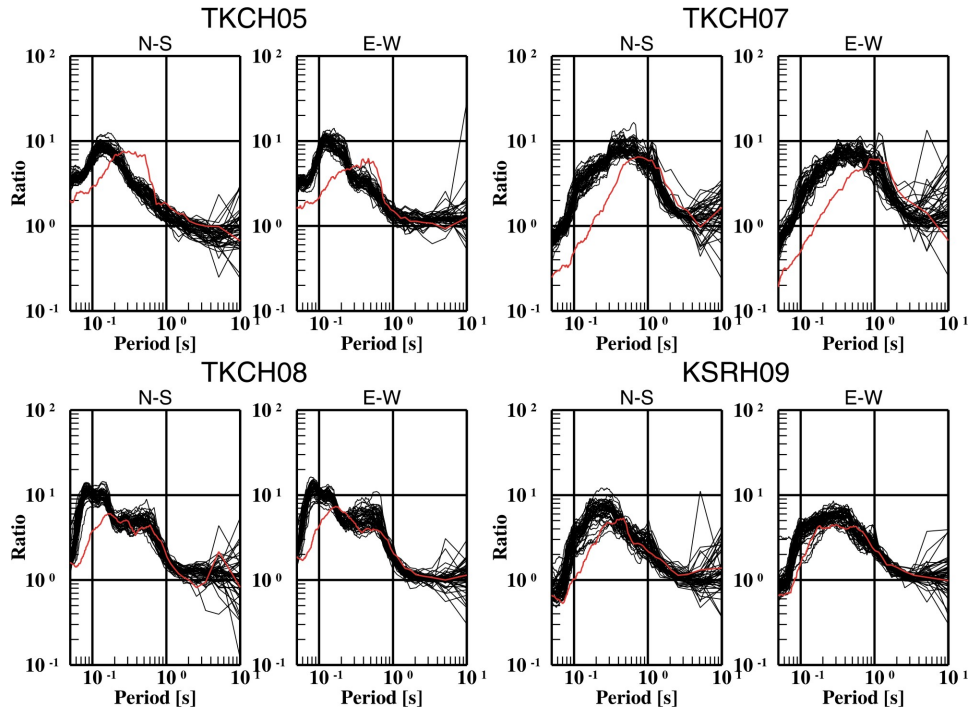
図 2.2.6-4 図 2.2.6-3(2) に示した KiK-net 観測点における地表と地中の観測記録のスペクトル比 (S波部分：地表/地中、赤線は十勝沖地震の本震記録、黒線はその他の地震記録)
