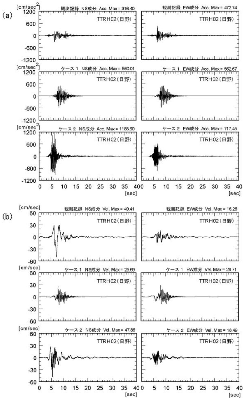
図2.1.3-3(1) 地中観測点における地震波形（観測波形、ケース1、ケース2）の比較（日野観測点；（a）：加速度波形 （b）：速度波形）
