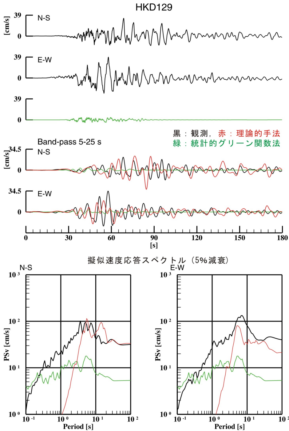
図 2.2.6-1(1) 平成 15 年 (2003 年) 十勝沖地震の観測記録と強震動計算結果の波形比較の例 (その 1 : 統計的グリーン関数法、理論的手法と観測記録との比較)
