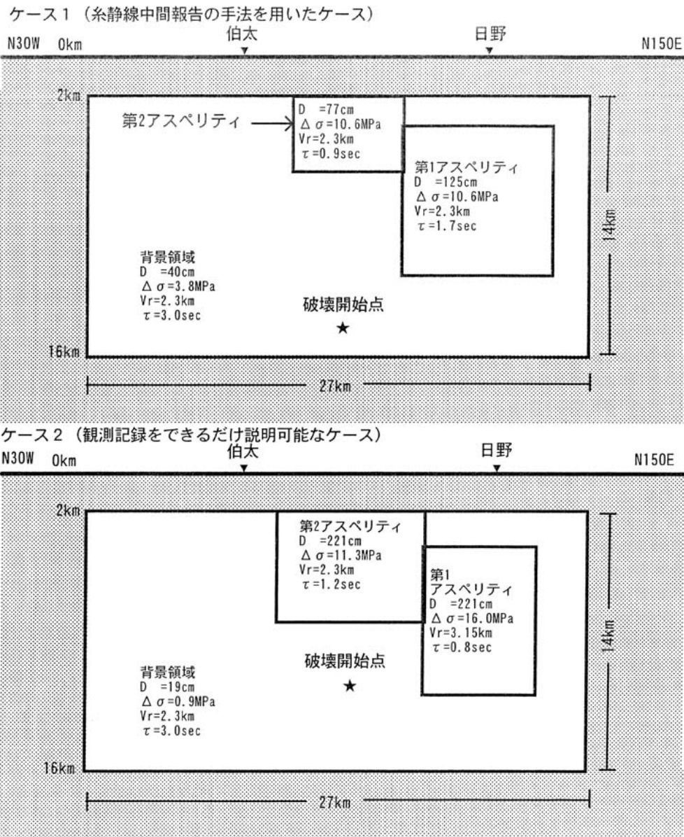
図2. 1. 3-2 鳥取県西部地震のアスペリティ位置図および主要なパラメータ
