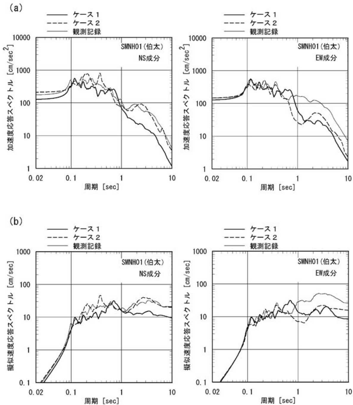
図2.1.3-4(2) 地中観測点におけるスペクトル（観測波形、ケース1、ケース2）の比較（伯太観測点；（a）：5%減衰加速度応答スペクトル、（b）：5%減衰擬似速度応答スペクトル）
