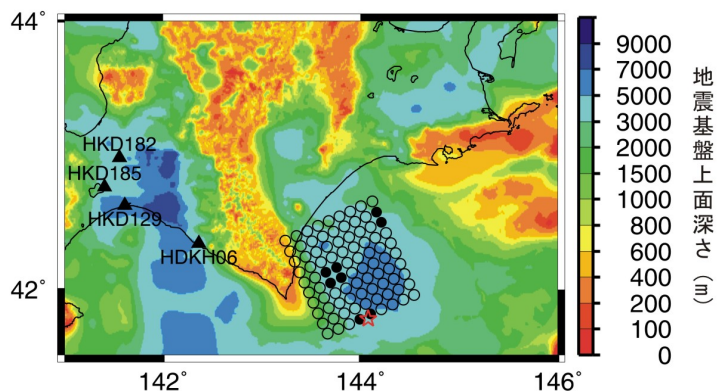
図 2.2.6-3(3) 平成 15 年 (2003 年) 十勝沖地震の観測波形記録と詳細法による計算波形との比較例 (つづき: 堆積層の厚い平野内の観測点)
