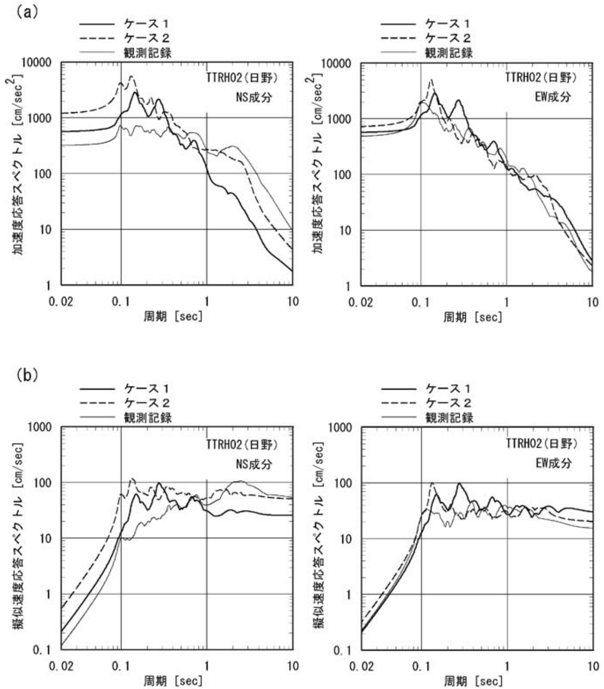
図2.1.3-4(1) 地中観測点におけるスペクトル（観測波形、ケース1、ケース2）の比較（日野観測点；（a）：5%減衰加速度応答スペクトル、（b）：5%減衰擬似速度応答スペクトル）
