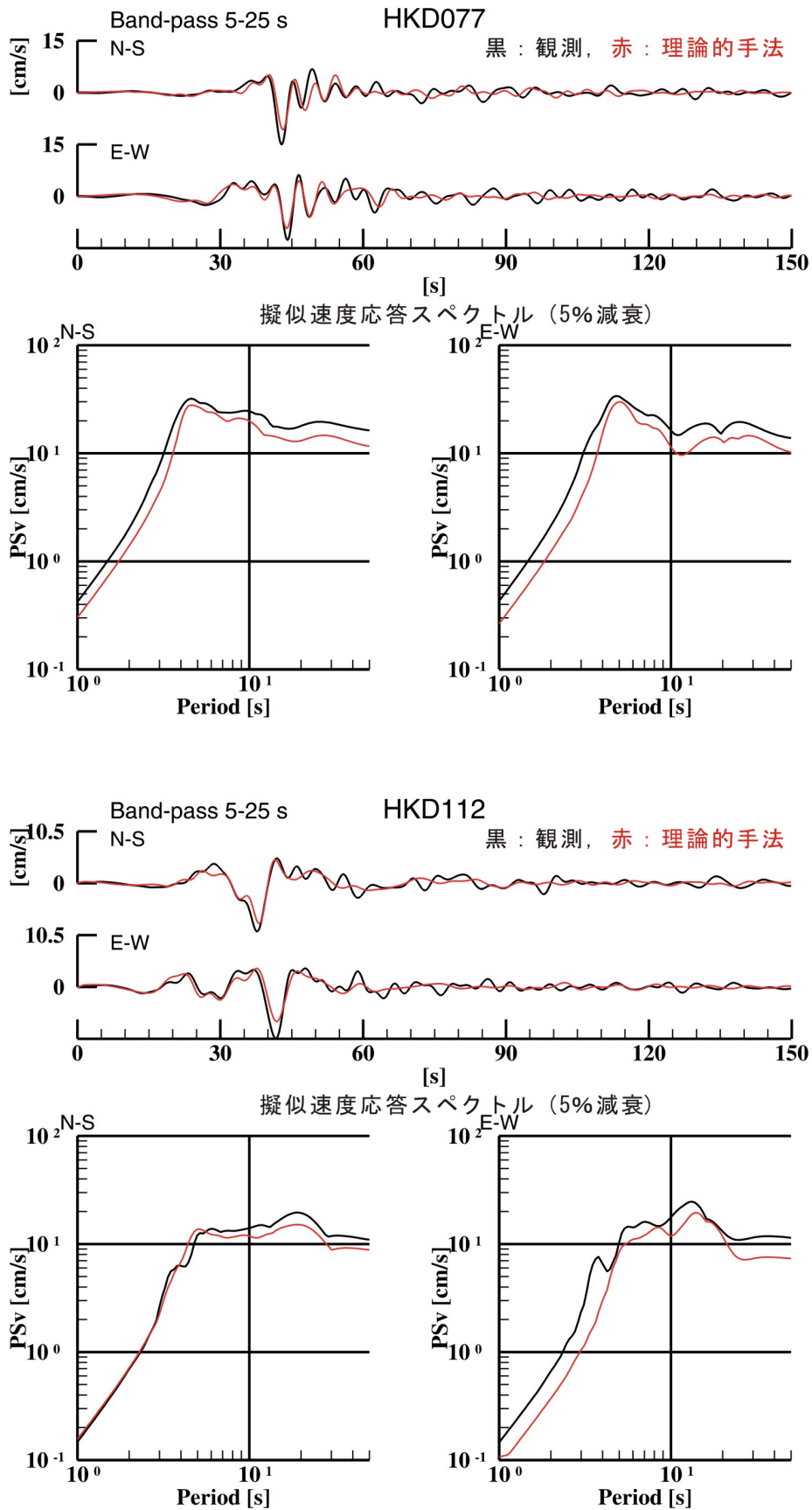
図 2.2.6-1(2) 平成 15 年 (2003 年) 十勝沖地震の観測記録と強震動計算結果の波形比較の例 (その 2 : 理論的手法と観測記録との比較、観測記録には、5 秒～25 秒のバンドパスフィルターを施している。)
