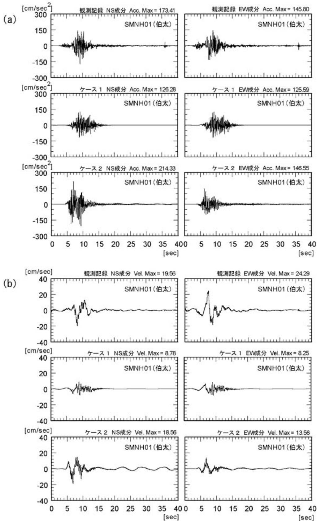
図2.1.3-3(2) 地中観測点における地震波形（観測波形、ケース1、ケース2）の比較（伯太観測点；（a）：加速度波形 （b）：速度波形）
